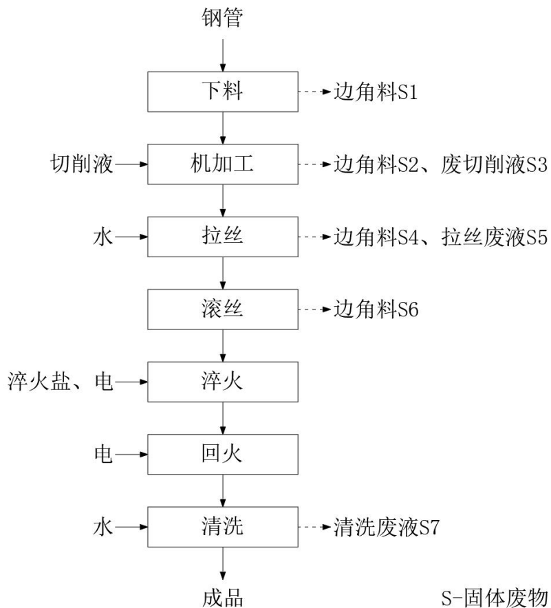
图 2.2-1 气弹簧配件制造工艺流程及产污环节图
