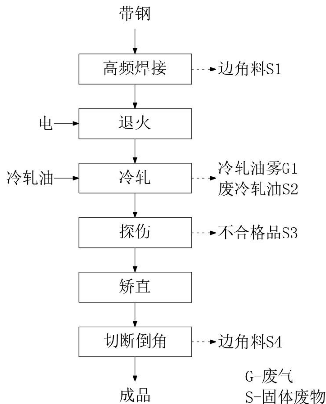
图 2.2-1 气弹簧及减震机配件制造工艺流程及产污环节图 生产工艺流程简述：
